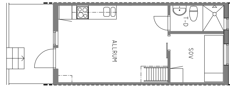
PLAN TYP B SKALA 1:50
