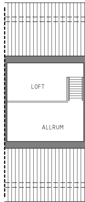
PLAN TYP A, LOFT SKALA 1:50
