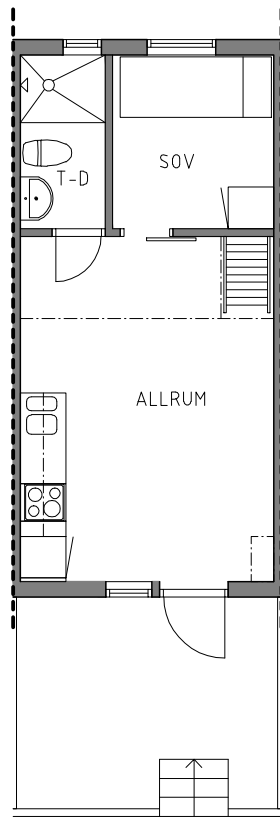
PLAN TYP A SKALA 1:50
